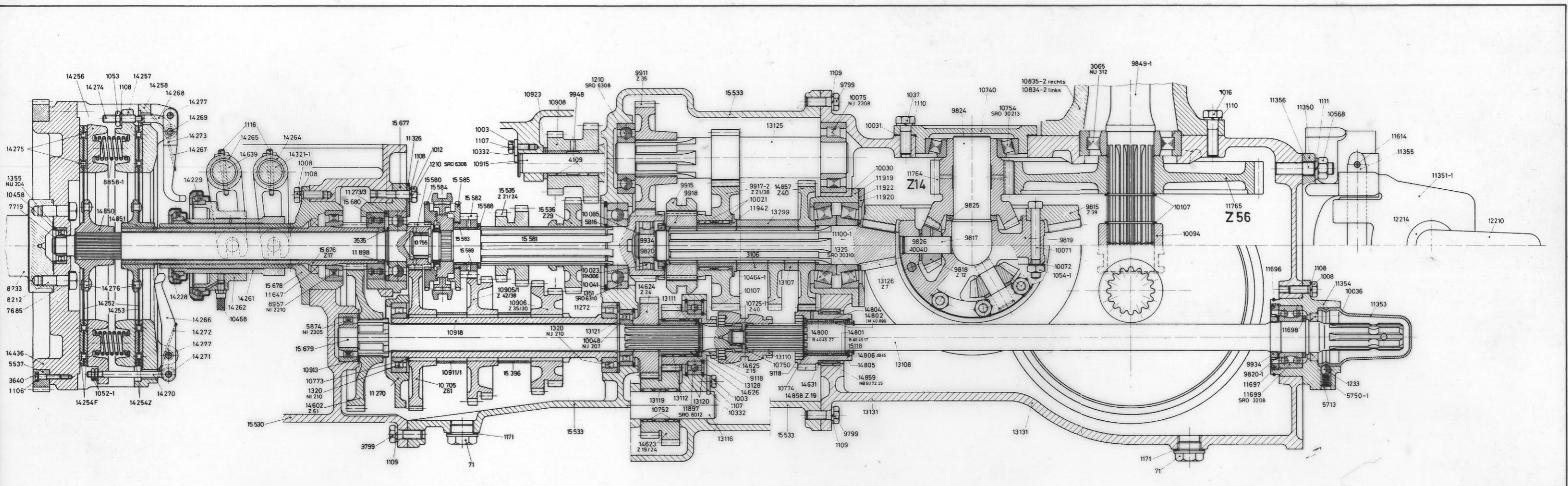
5200 Getriebelängsschnitt T-6200 neue Ausführung (grosse Kupplungs-Lamellenmuffe) Z-790
