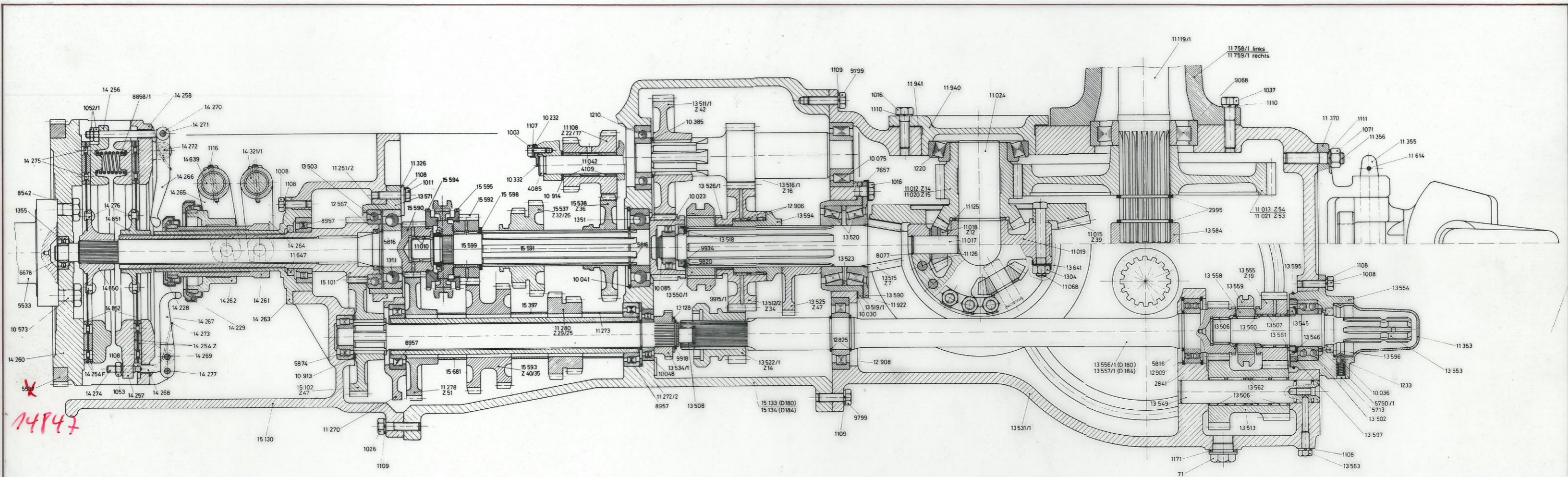
Getriebelängsschnitt 7700 / T-9200
