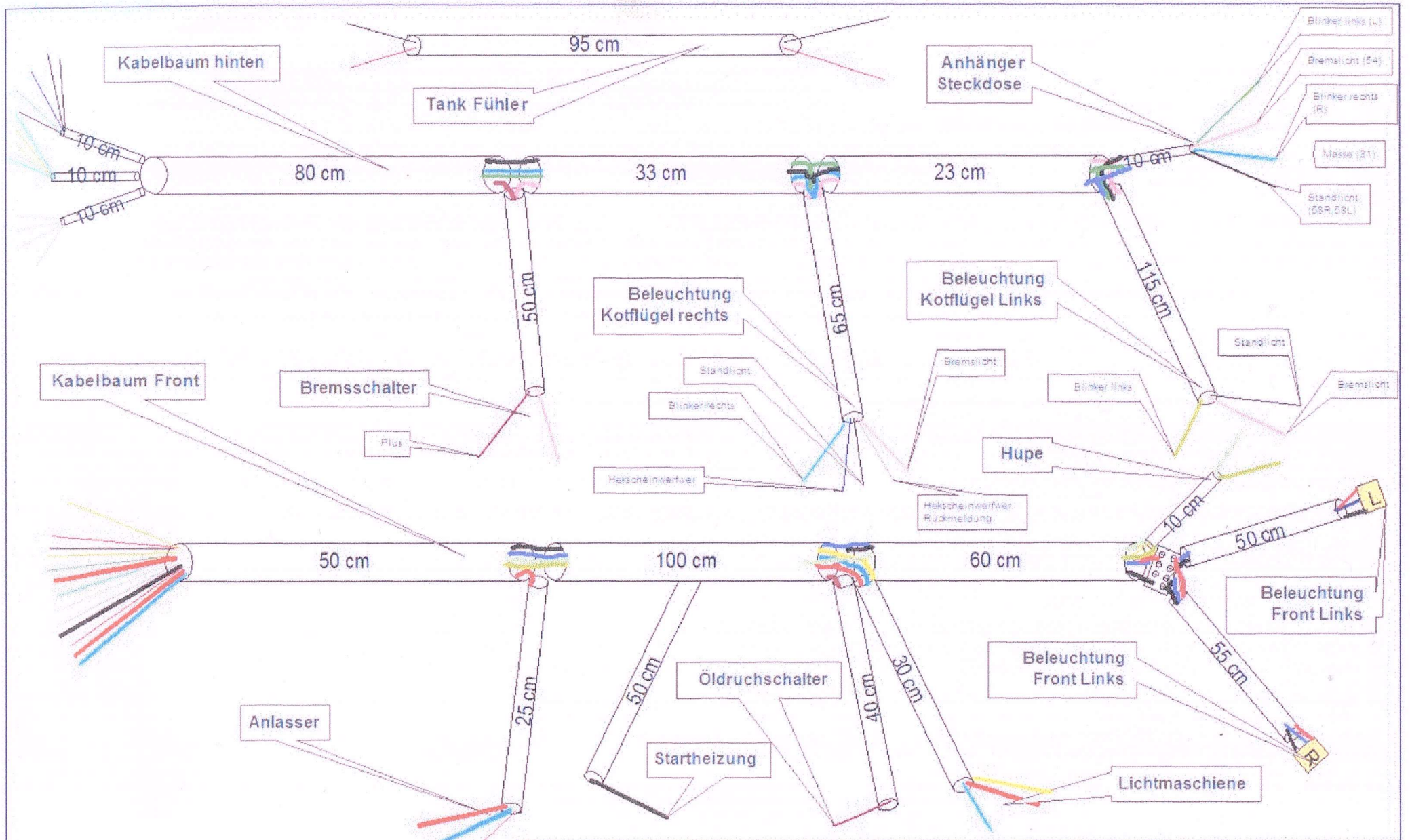
Hürlimann Kabelbaum D115 - D 310
